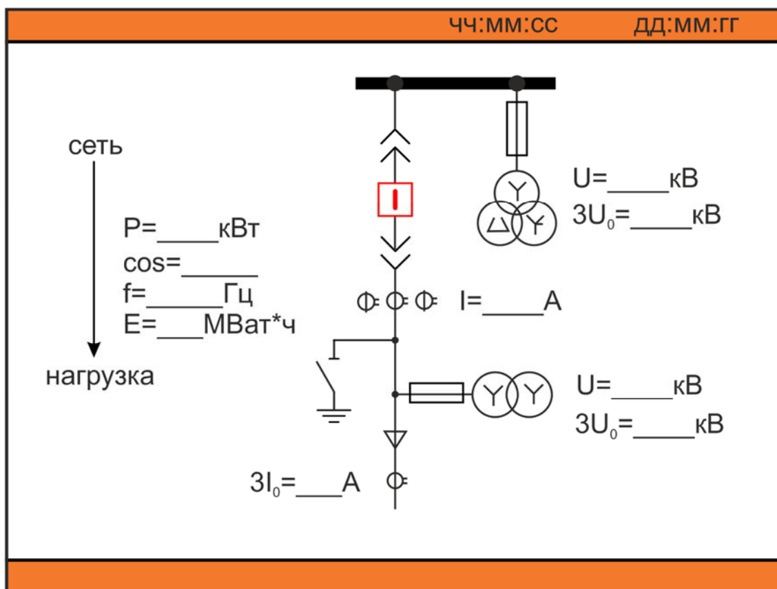
Рис.2.4.1. Мнемосхема терминала РЗА
