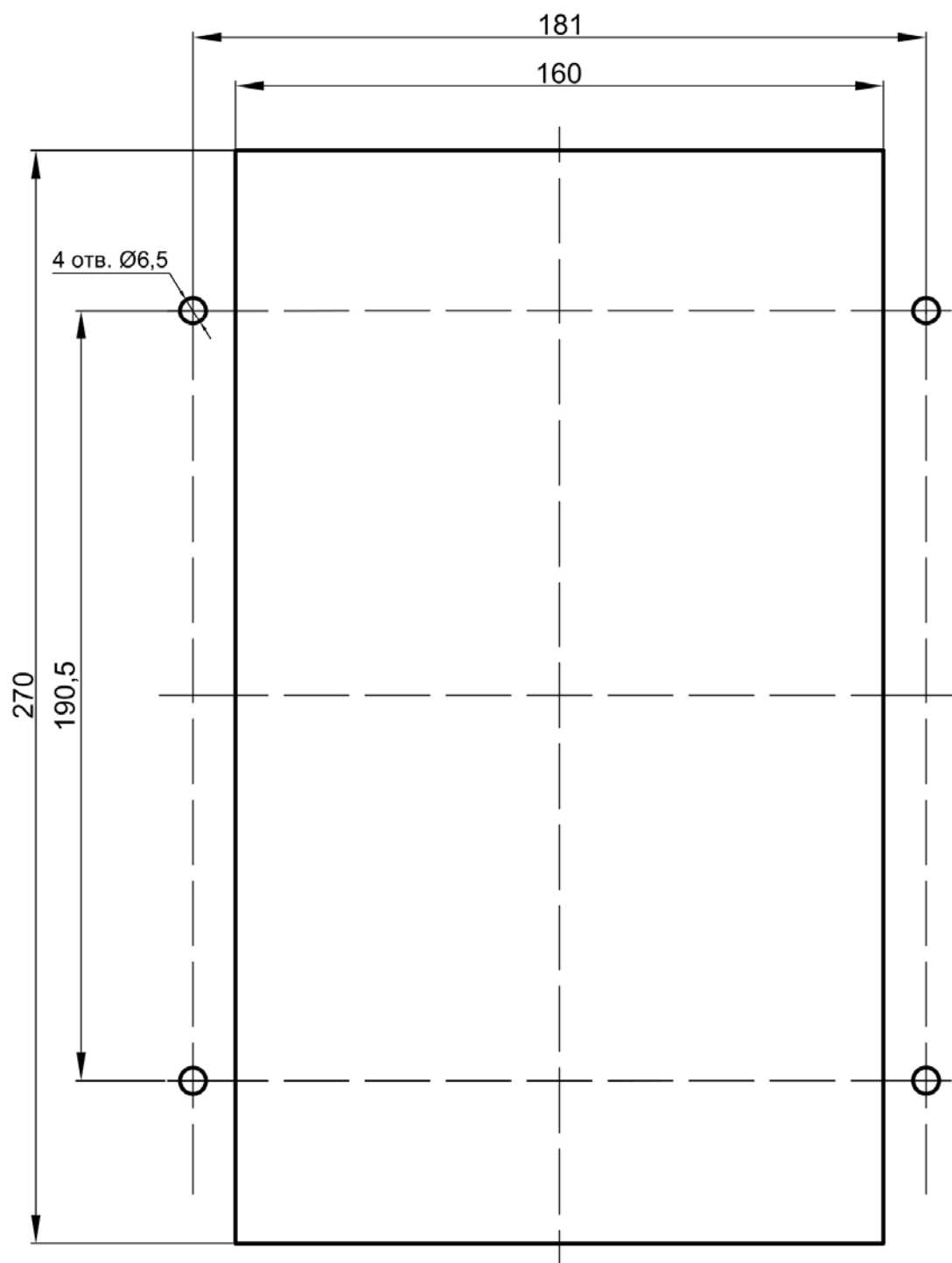
Рис. П2.5. Монтажные отверстия для установки терминала «МИР 100»
