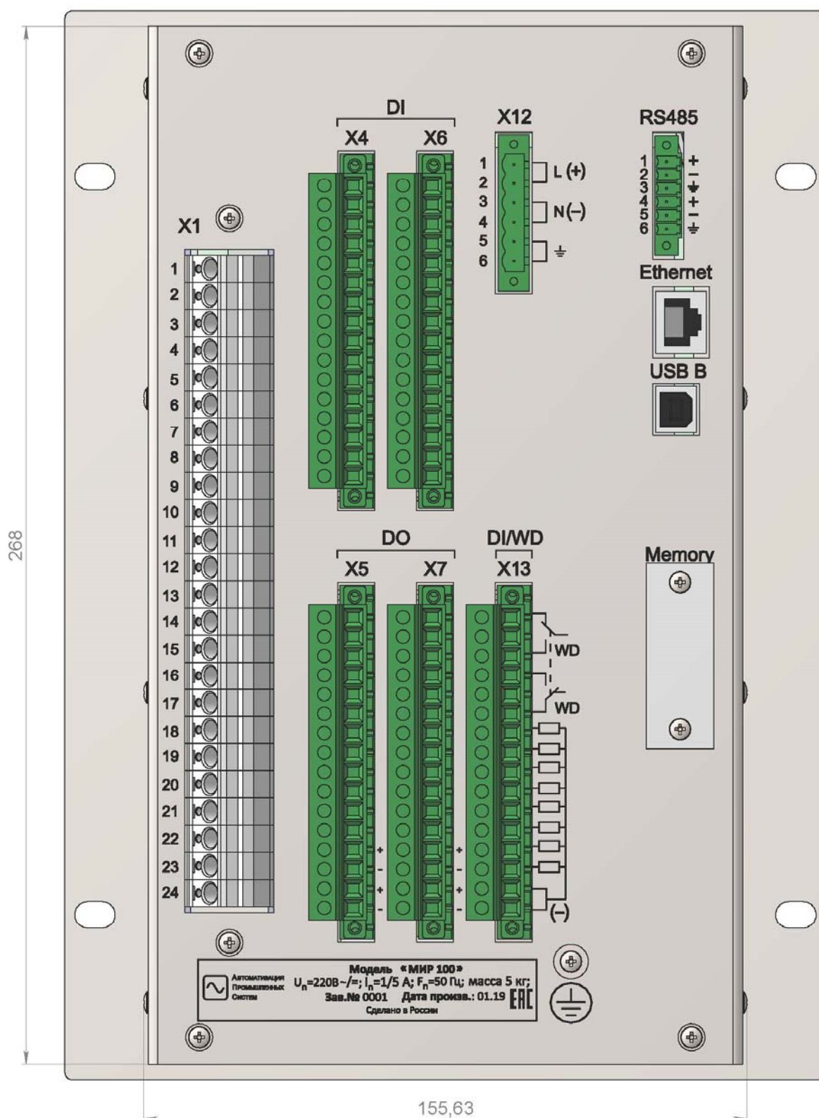
Рис. П2.2. Внешний вид задней части терминала «МИР 100».
