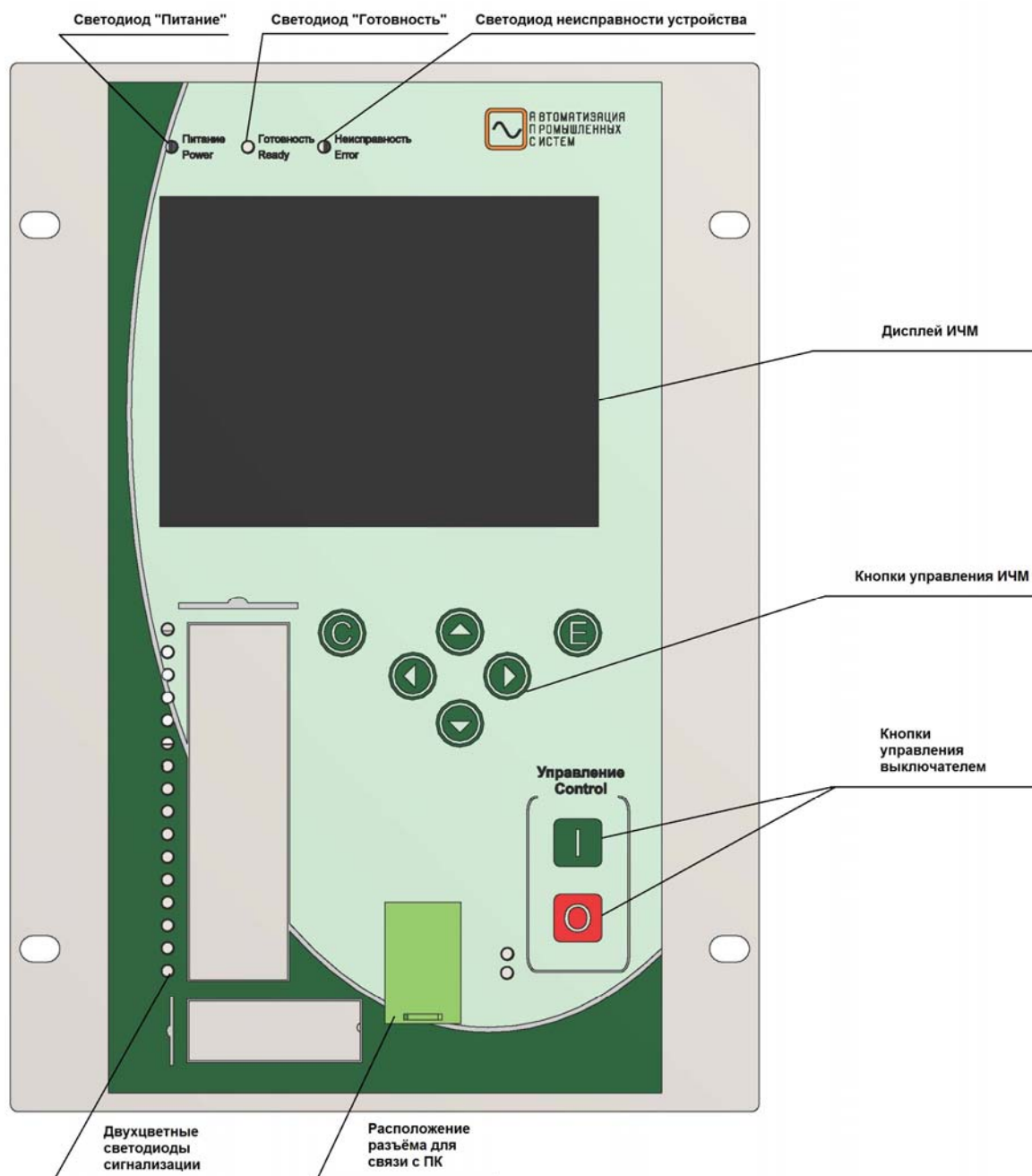
Рис. П2.6. Расположение элементов управления и индикации терминала «МИР 100»
