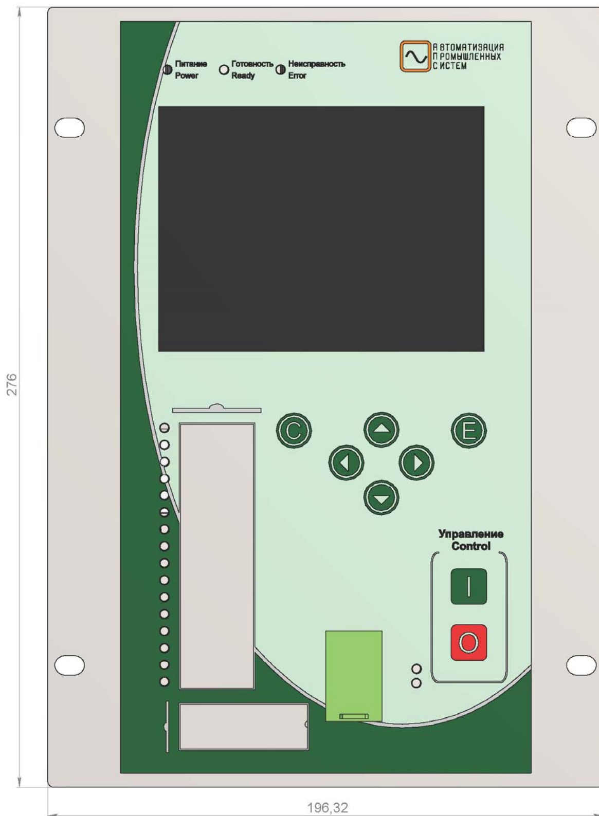
Рис. П2.1. Внешний вид передней части терминала «МИР 100»
