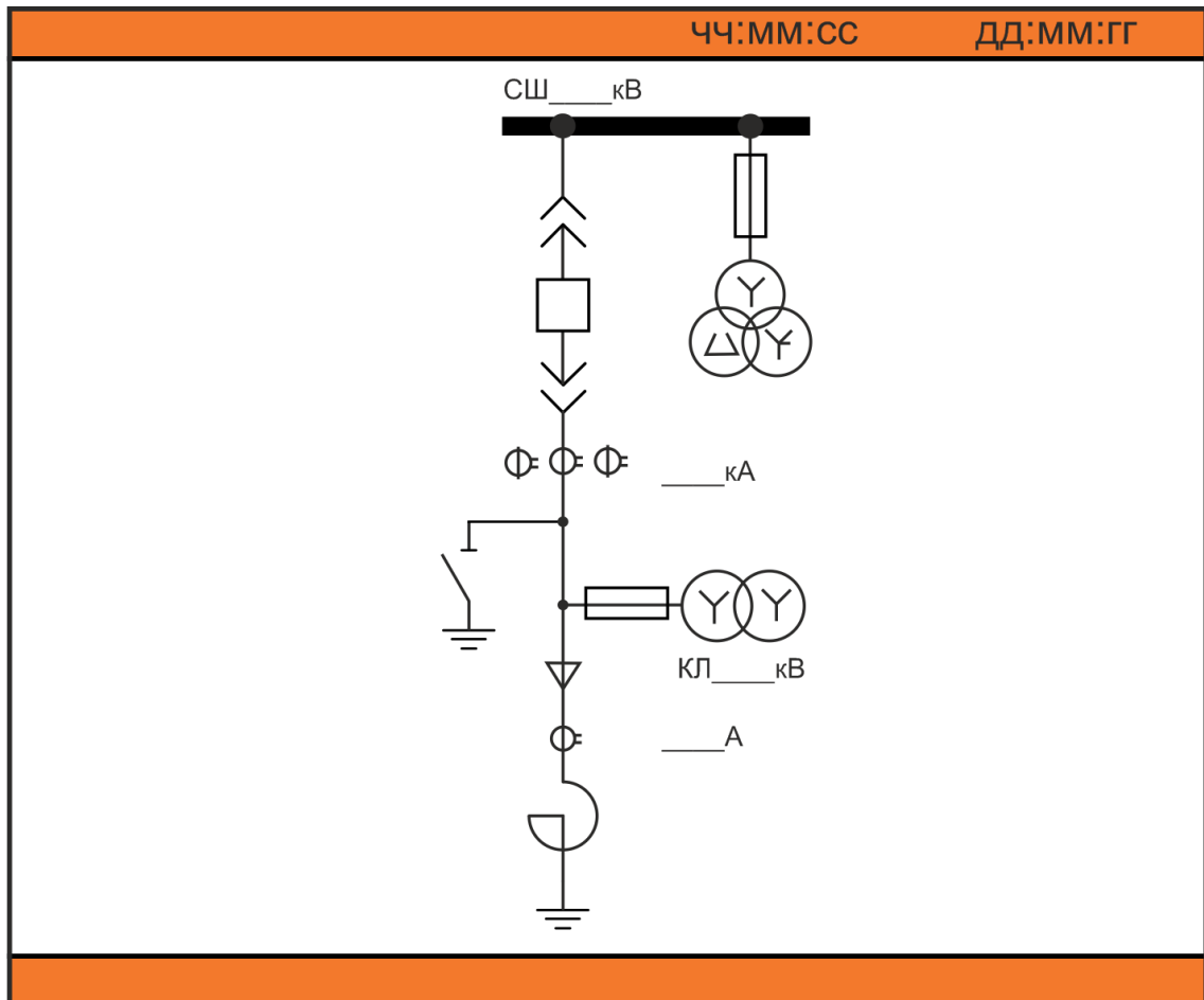
Рис.2.4.1. Мнемосхема терминала РЗА
