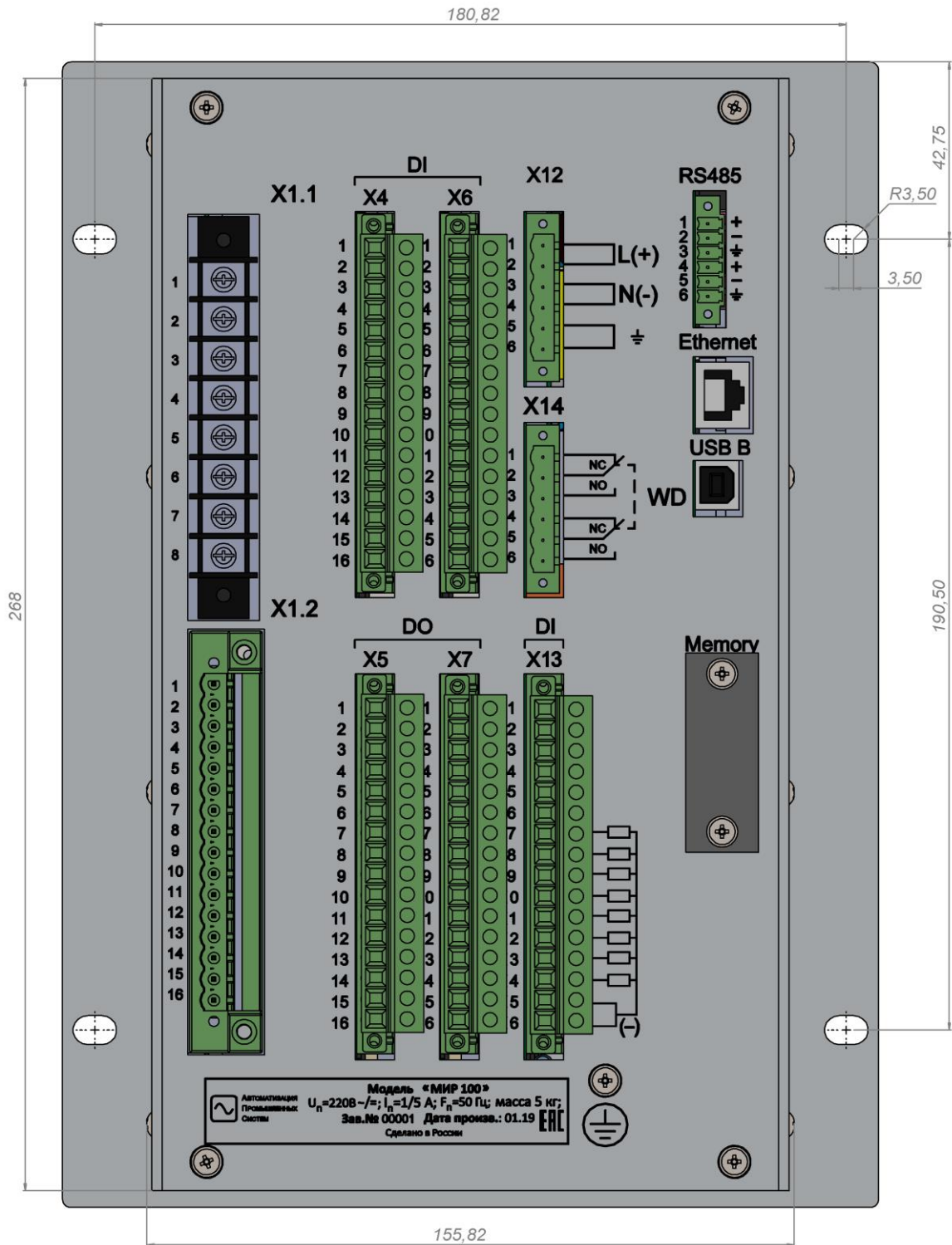
Рис. П2.2. Внешний вид задней части терминала «МИР 100».
