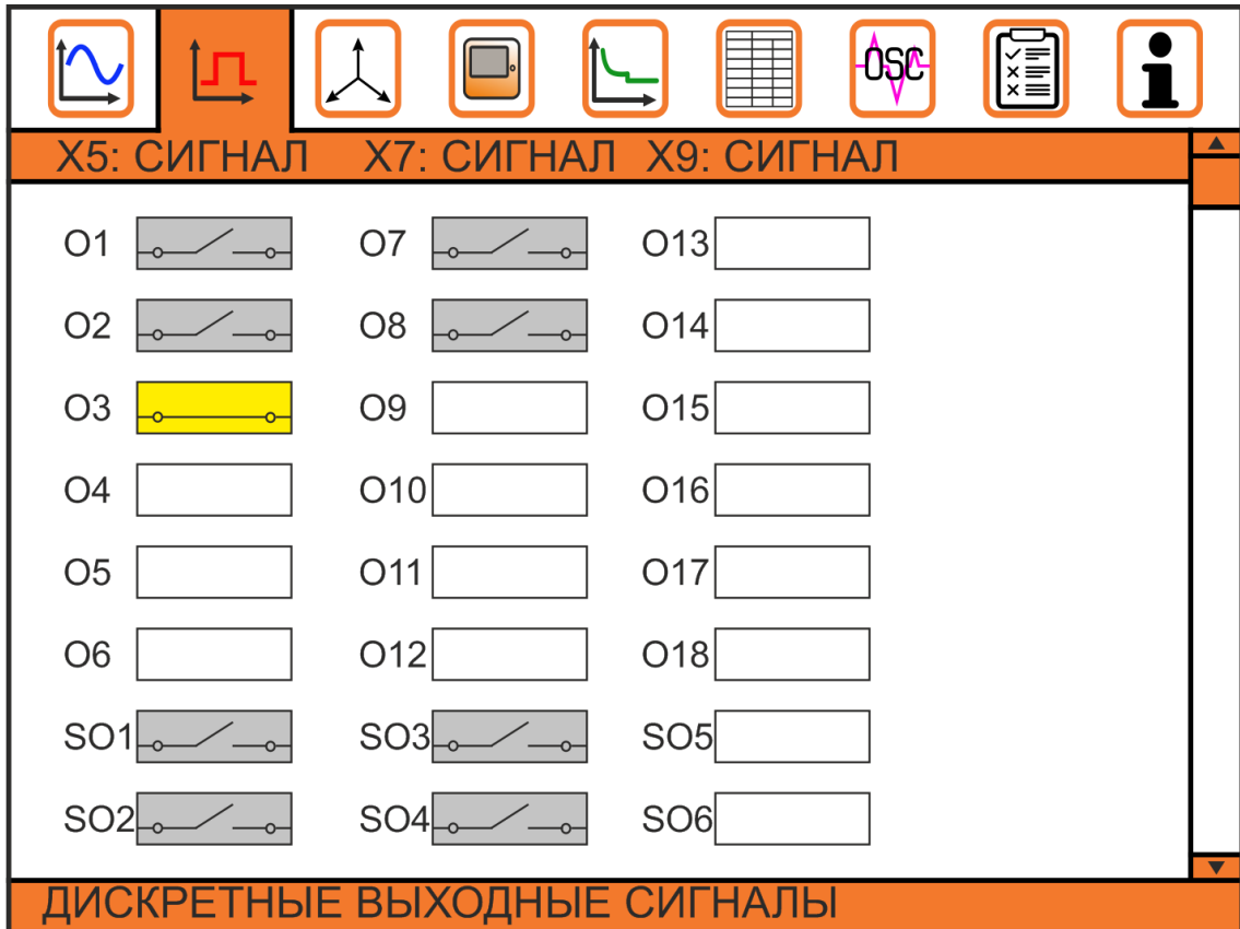
Рис. 2.4.6. Окно вкладки «Дискретные выходные сигналы», отображение по блокам
