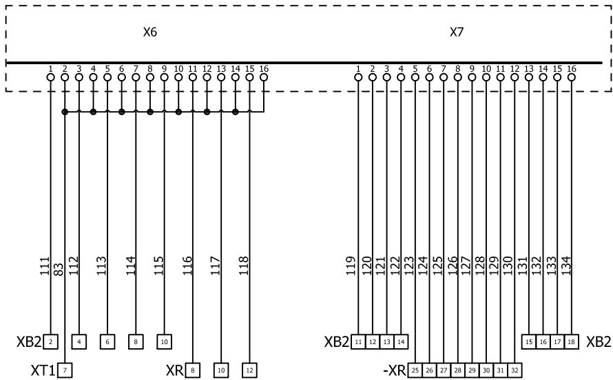
БЛОК Е5 ВВОД2
