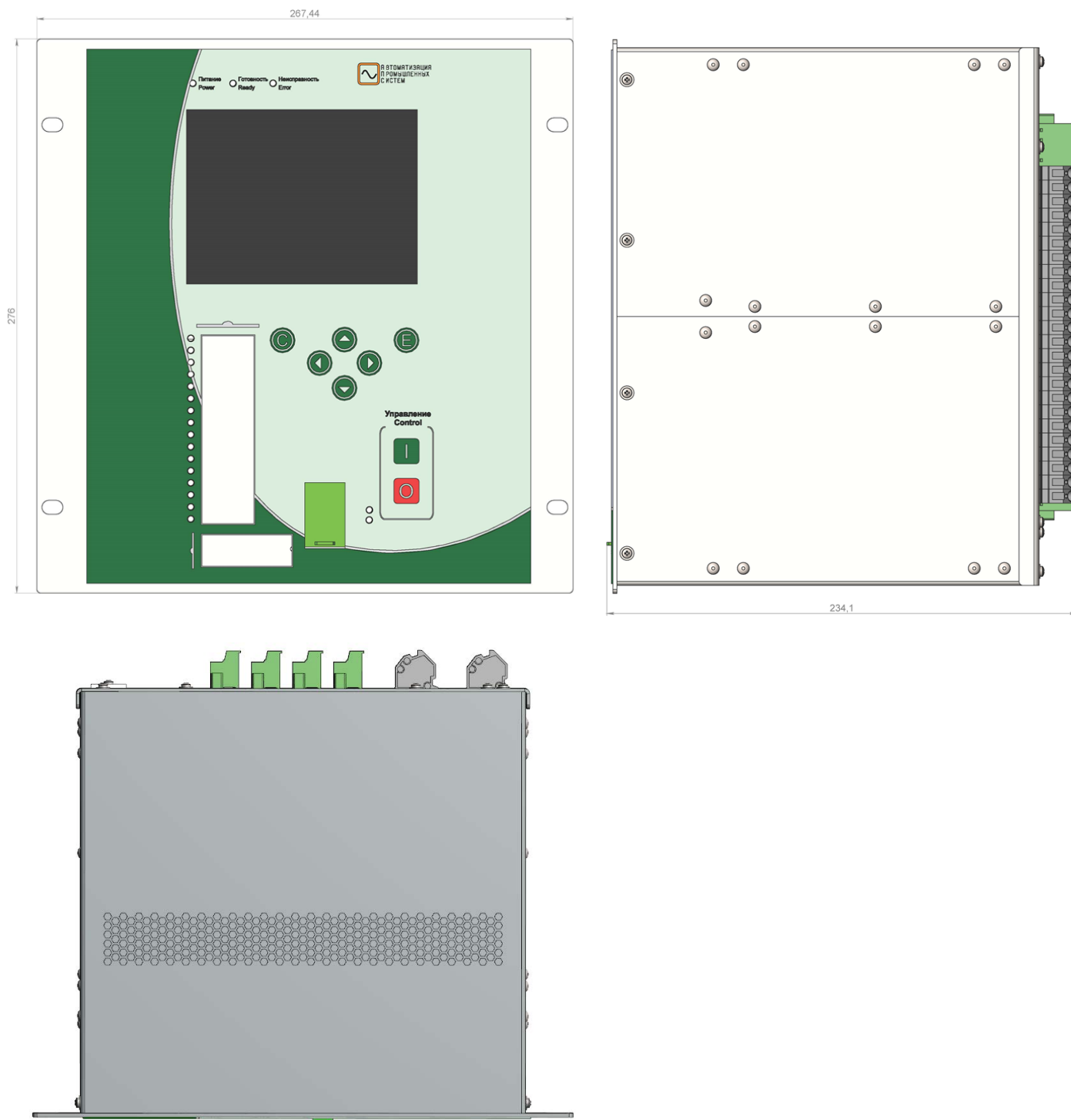
Рисунок Б.1 – Терминал серии БАВР_10_АПС-2-2-2022
