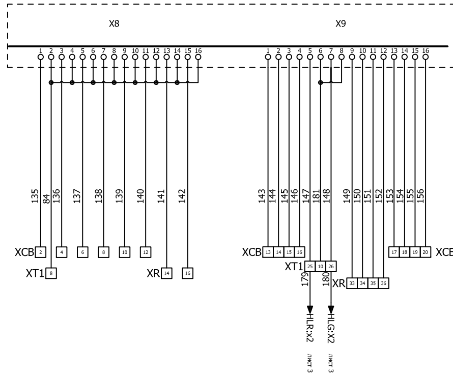
БЛОК Е6 СВ
